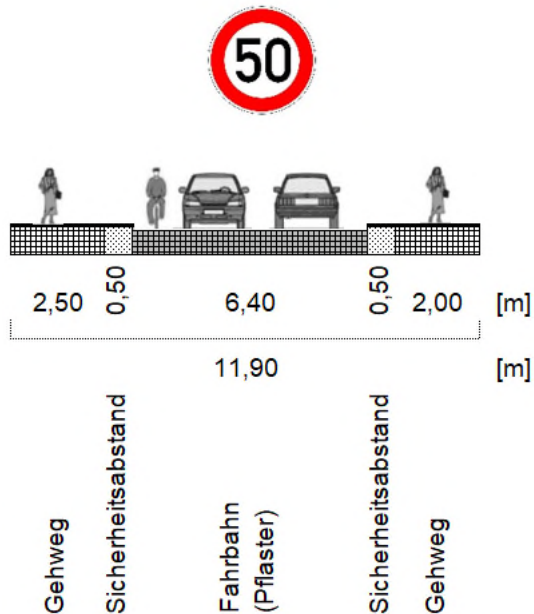
Abbildung 7-1: Vergleich der Querschnitte in der Beethovenstraße
